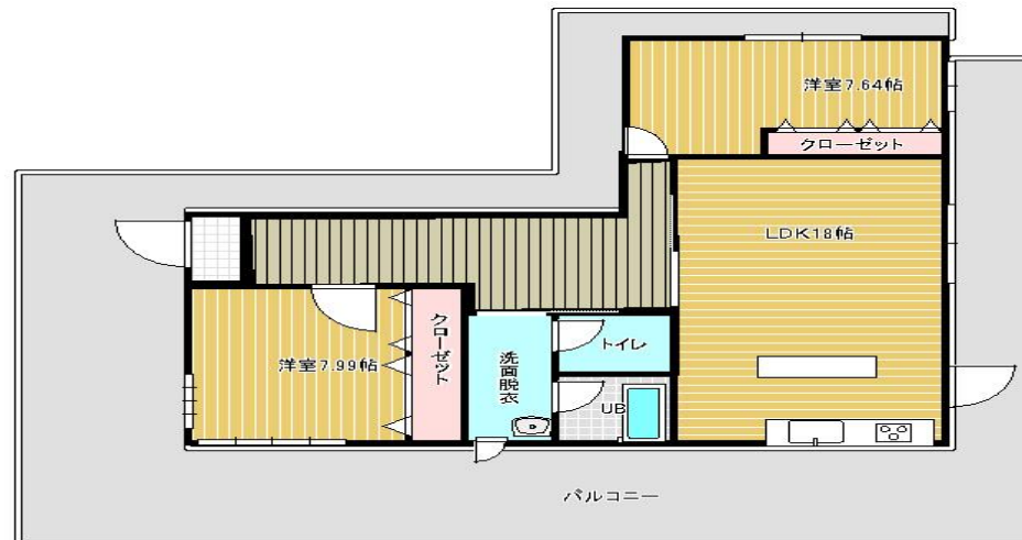
【間取り図】
